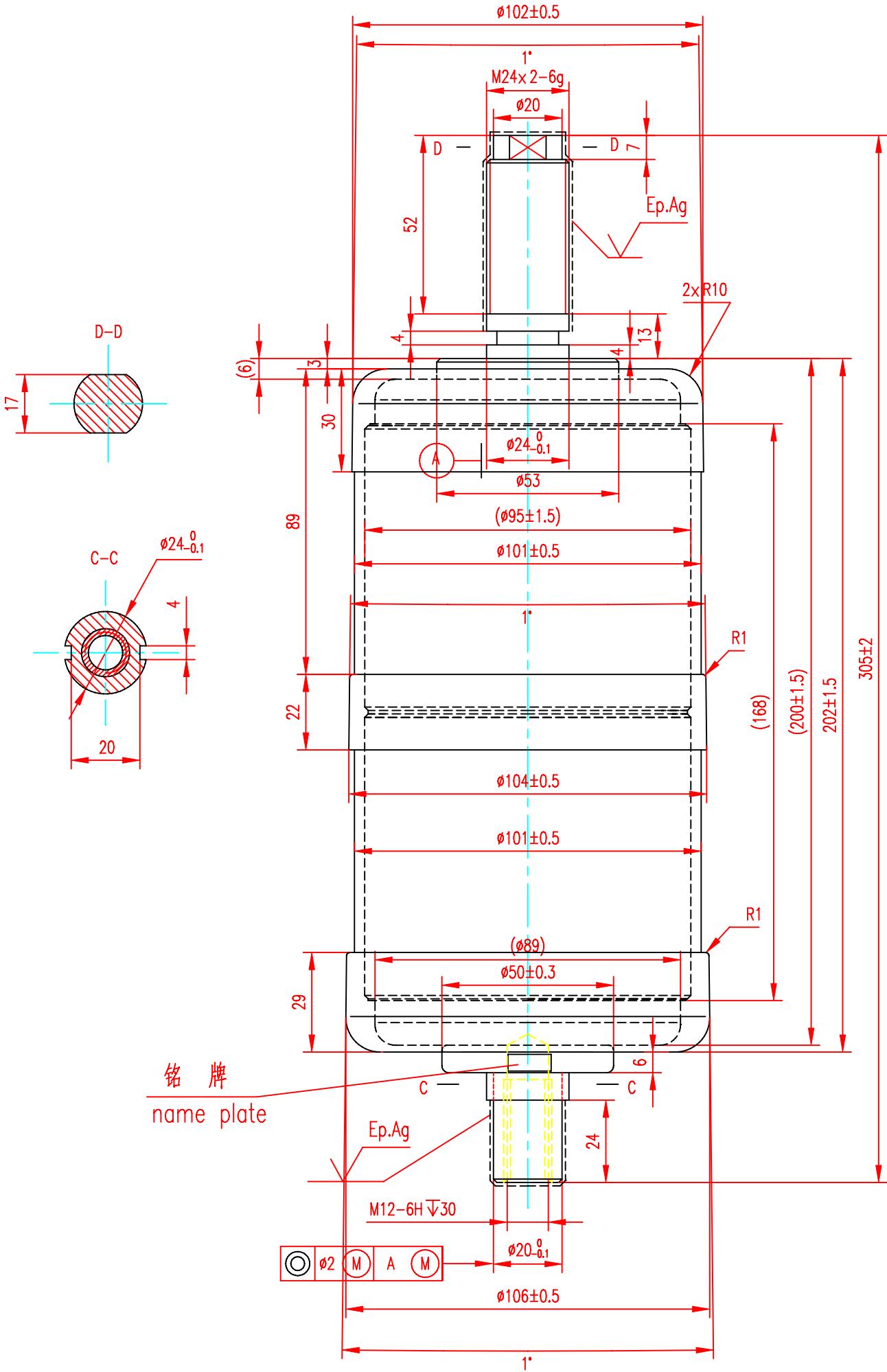
图1 DB3.393.094WX-G
